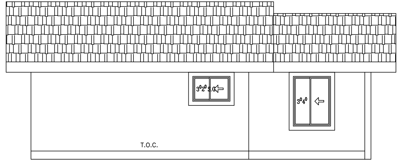
RIGHT SCALE: 1/4" = 1'
