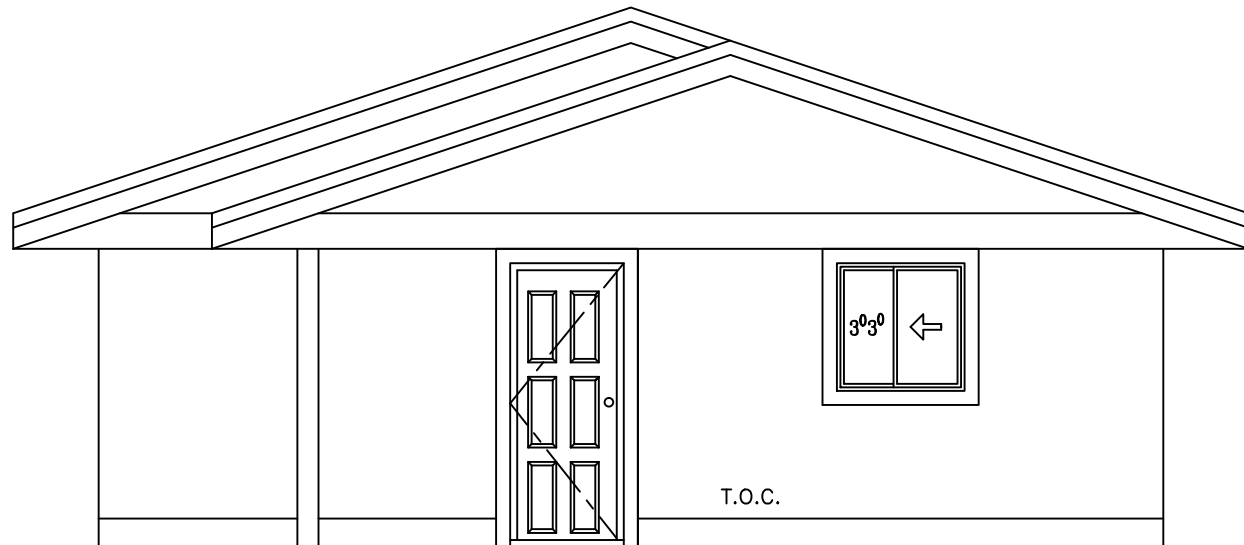
REAR SCALE: 1/4" = 1'
