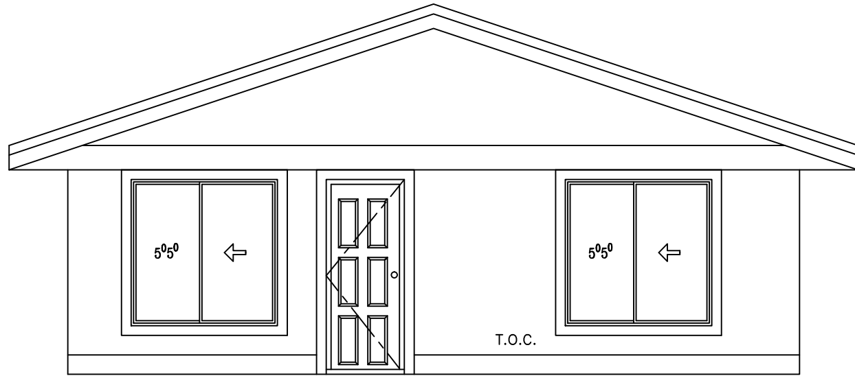
FRONT SCALE: 1/4" = 1'
